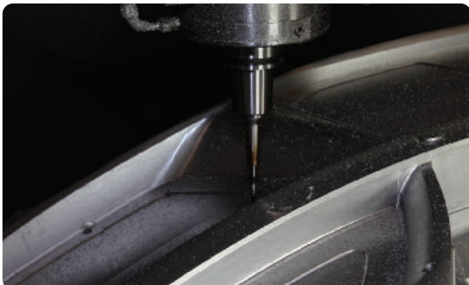
Präzisionsherstellung von PU-RIM Spritzgusswerkzeugen für Qualitäts-Serienfertigung. High-precision injection mold tooling enables quality volume production in PU-RIM.
